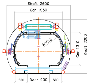
MRL 2:1 1000kg
