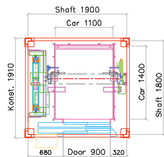
MRL 2:1 630kg
