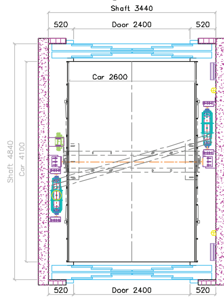
HDR 2:1 3.000kg
