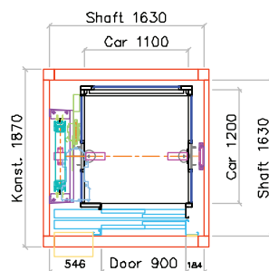
MRL 2:1 480kg
