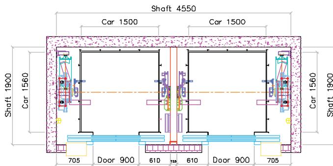
MRL 2:1 1000kg
