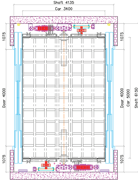
HDR 2:1 10.000kg
