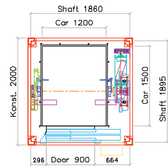
MRL 2:1 800kg
