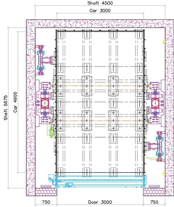
HDR 2:1 4.000kg
